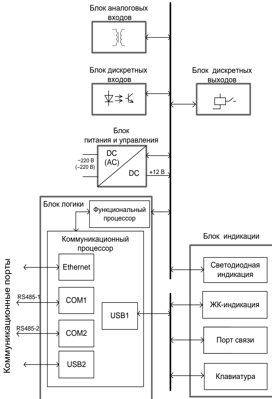
Рисунок В.1 – Базовая 1) блок-схема терминалов типов ЭКРА 2Х1(А), ЭКРА 2Х2(А), ЭКРА 2Х3(А), ЭКРА2Х7(А)
