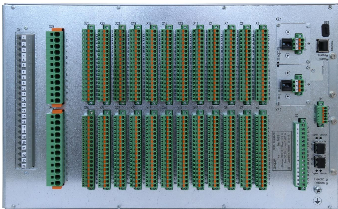
Рисунок Б.1 – Пример внешнего вида задней панели терминала
